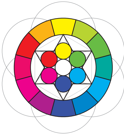
La Graine de Vie et les douze couleurs de la roue chromatique plus le blanc et le noir soit 14 couleurs en tout
